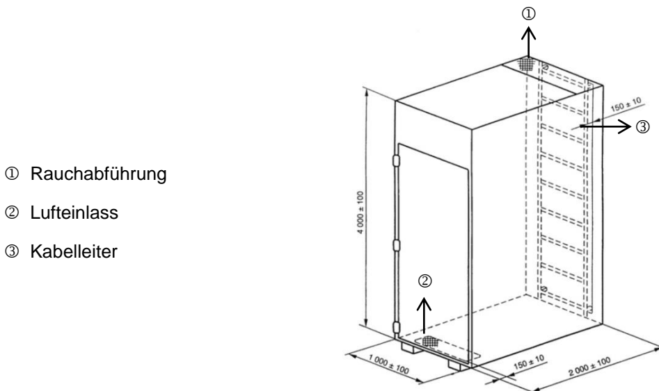
Abbildung 1: Kabelschacht nach EN 60332-3-10 Figure 1: Cable duct according to EN 60332-3-10
