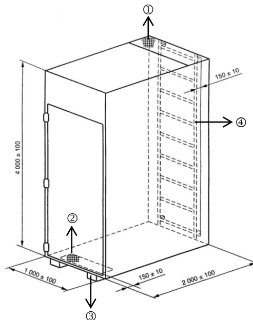
Abbildung 1: Kabelschacht nach EN 60332-3-10 Figure 1: Cable duct according to EN 60332-3-10
