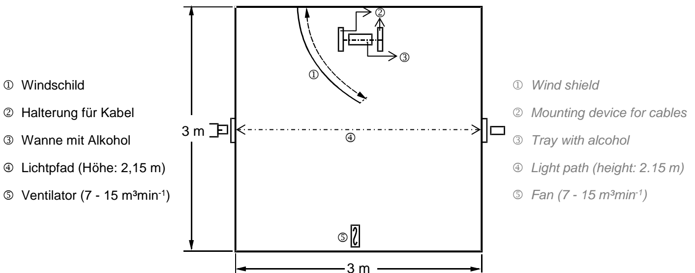
Abbildung 4: Schematische Darstellung der Prüfkammer (Cube) Figure 4: Diagram of the test chamber (cube)
