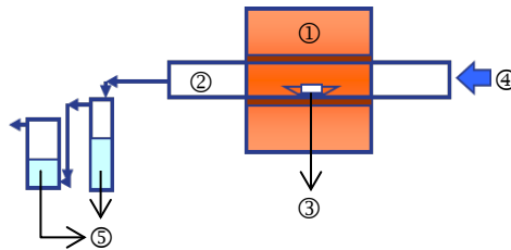
Abbildung 6: Prüfapparatur nach NF X 70-100 Figure 6: Test apparatus according to NF X 70-100
